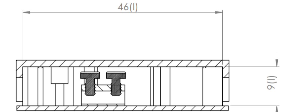
Sección / Section L-L
