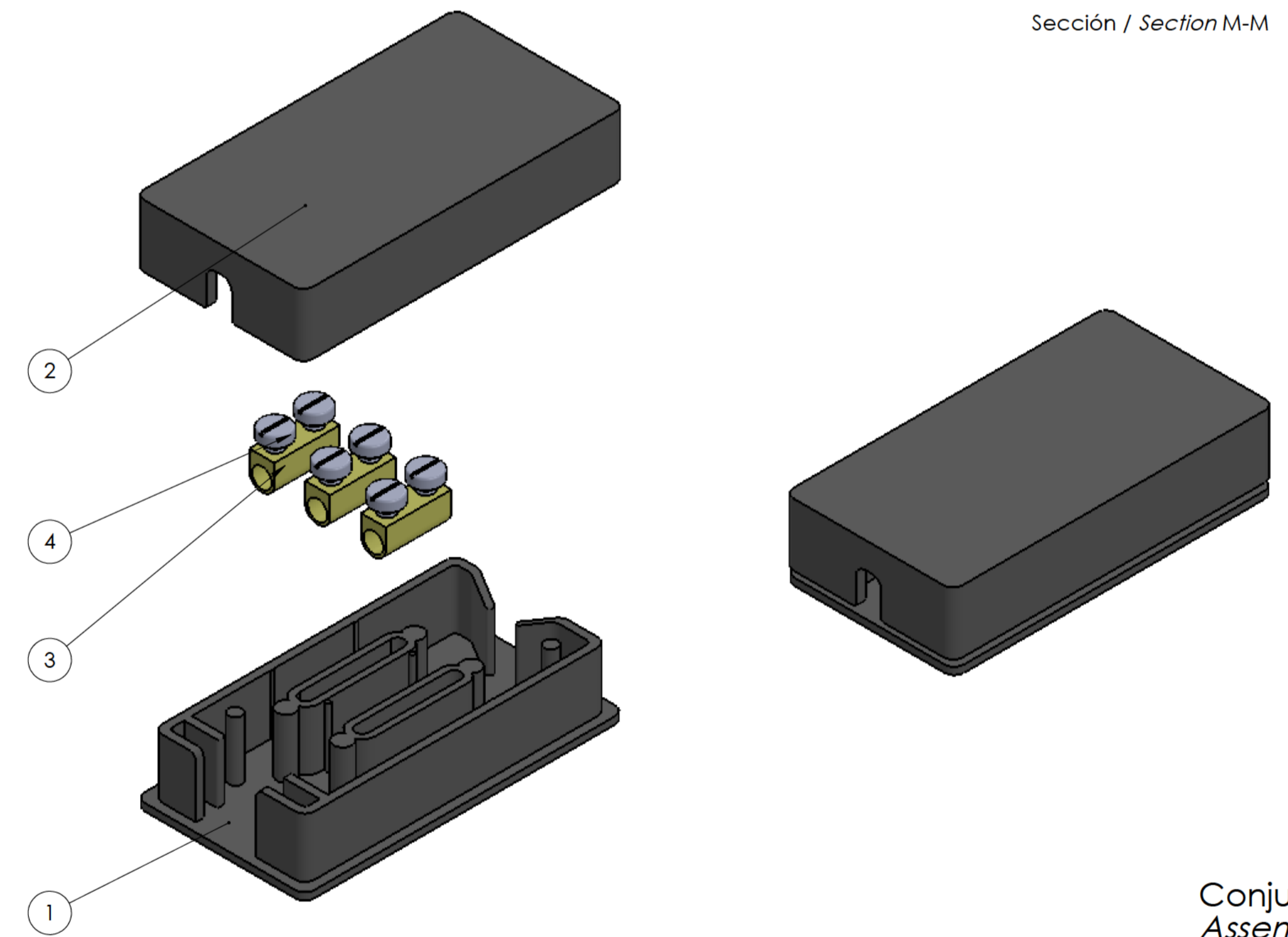
Sección / Section M-M
